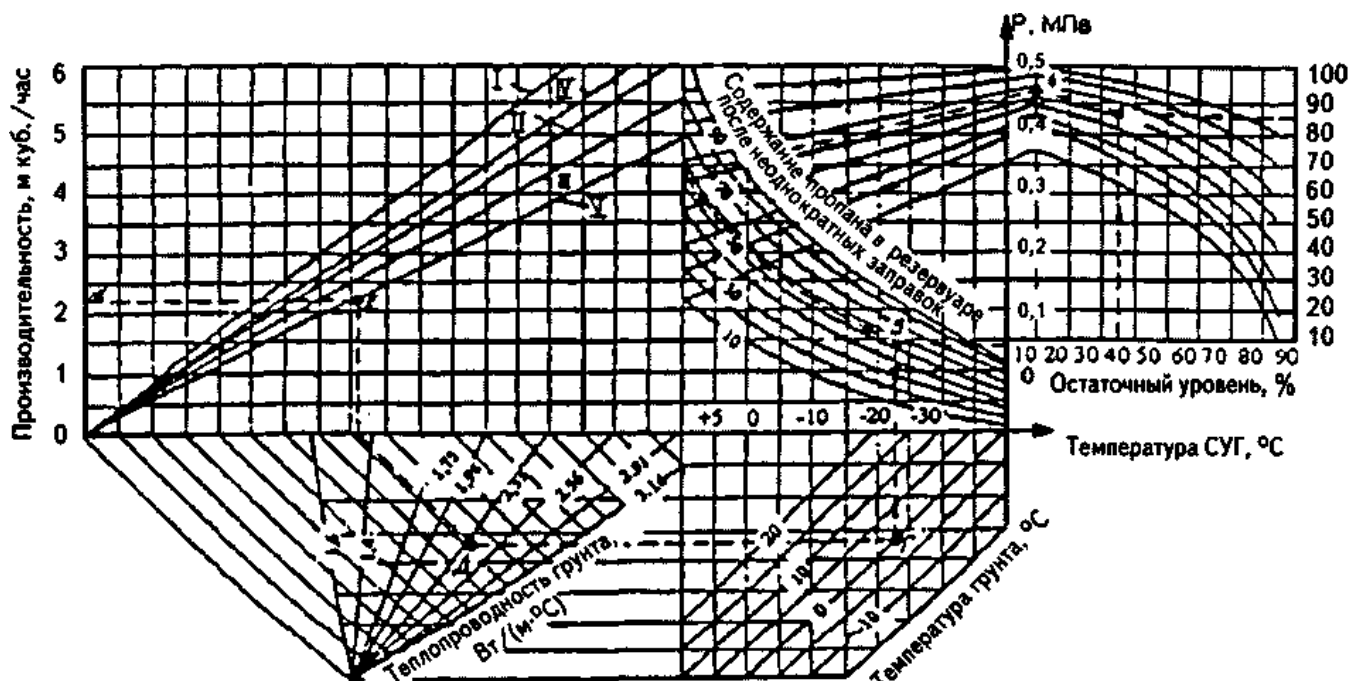
Номограмма для определения производительности резервуара сжиженного газа вместимостью 2,5 и 5 м³ (подземного)
